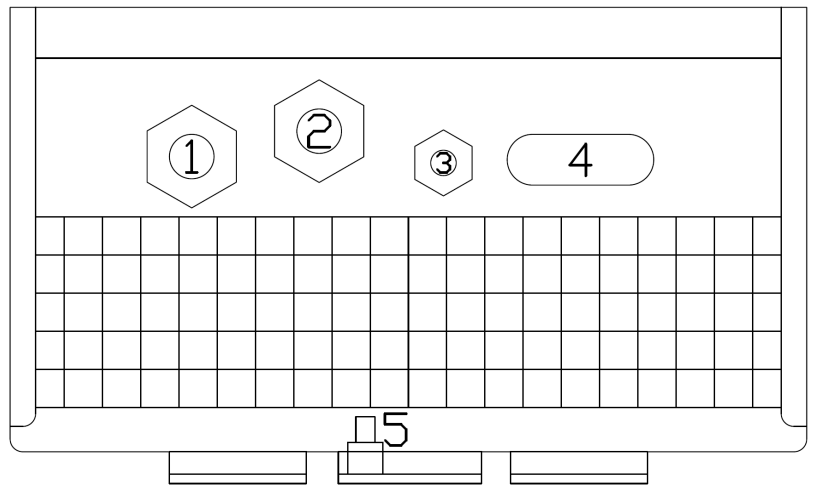
Figura 6 Vista dal basso dell'armadio in cui sono visibili gli ingressi dei cavi: modelli a due uscite
