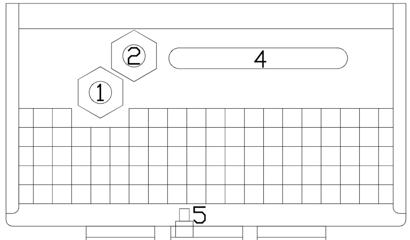
Figura 2 Vista dal basso dell'armadio in cui sono visibili gli ingressi dei cavi: modelli a tre uscite
